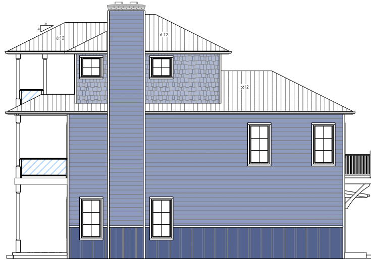
RIGHT ELEVATION
