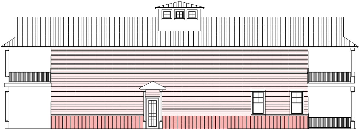
RIGHT ELEVATION
