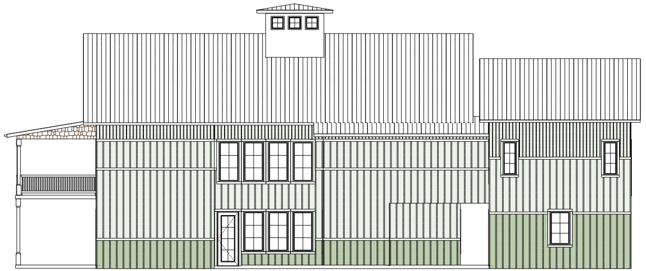
RIGHT ELEVATION
